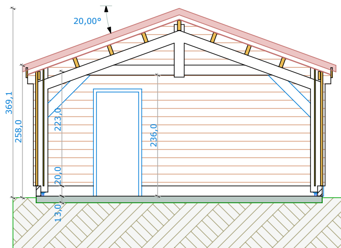
SNEDE A
